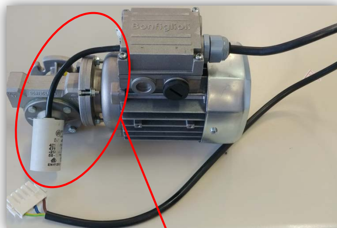
Condensatore pre – modifica integrato nel motoriduttore
